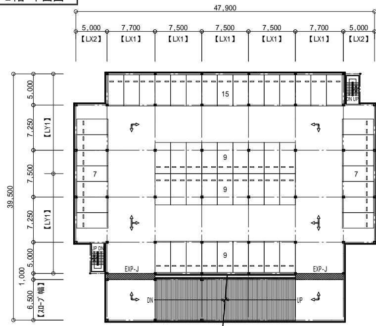
2階 平面図
