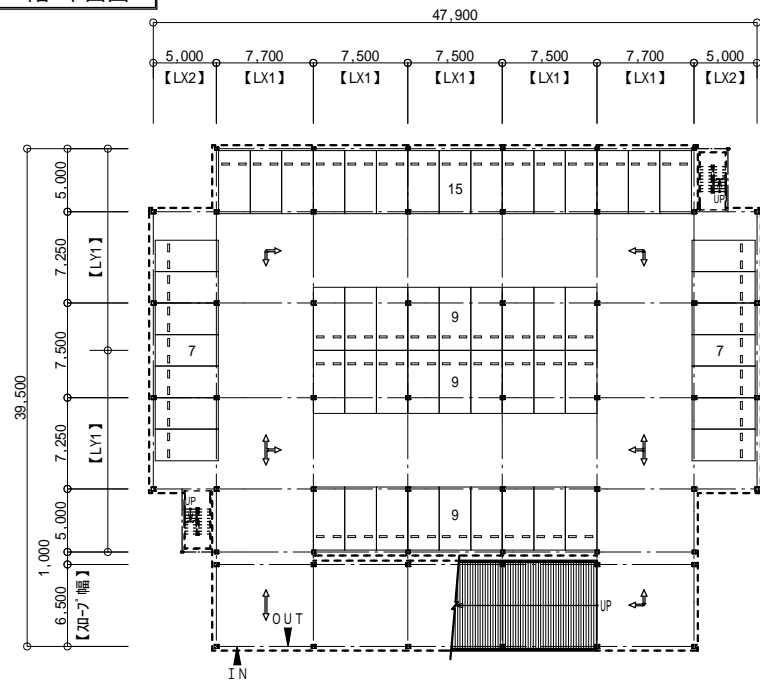
1階 平面図
